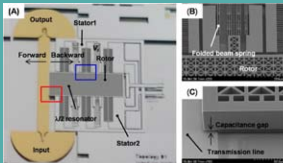
Fig.1 Resonador de microondas MEMS
